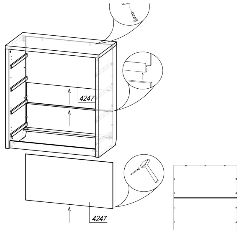
Схема расположения фиксаторов задней стенки ДВП
