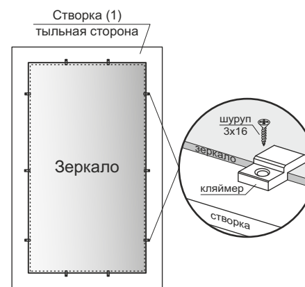
Рис.1 Вид сзади
