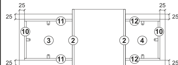
Рис.2 Крепление основания Вид снизу
