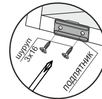
Рис.2 Крепление основания Вид снизу
