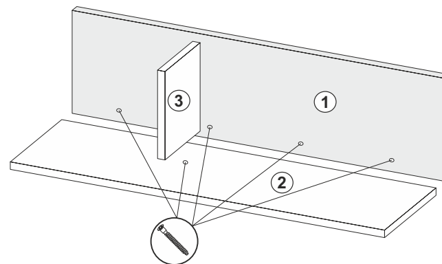
Рис.2: Вид спереди
