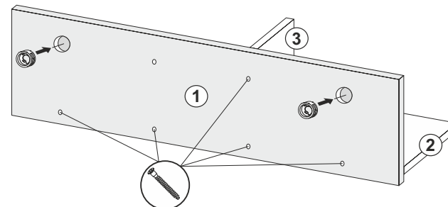
Рис.2: Вид спереди
